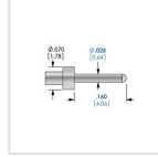
STP-25J160-3R
