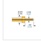
STP-25J100-3G
