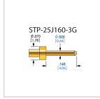
STP-25J160-3G
