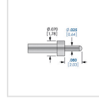
STP-25J080-3R
