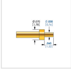
STP-25J100-3R
