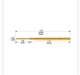
SPR-25W-3
