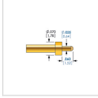
STP-25J140-3R
