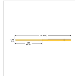
LTR-1W-2LL
