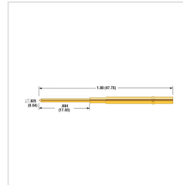
LTR-1W-2L
